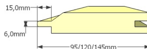
ENKELFASSPONT
