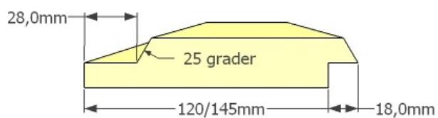
FALSAD SPÅRPANEL
