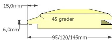
DUBBELFASSPONT
