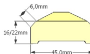
LOCKLÄKT
