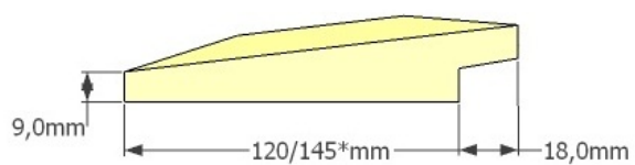
FJÄLLPANEL
